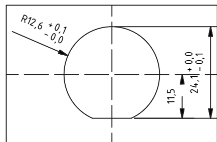
Frontplattenausschnitt
